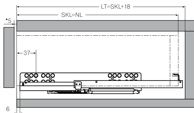
Присадка направляющих Push-to-open
