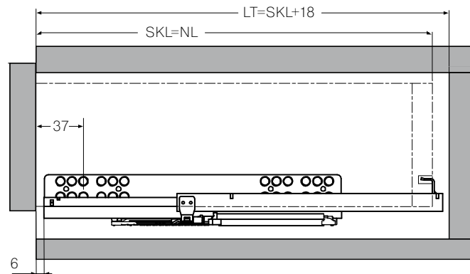
Присадка направляющих с/без доводчика
