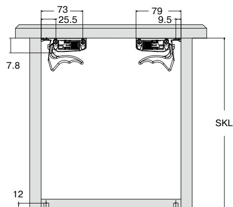
Присадка дна ящика с направляющими под фиксатор
