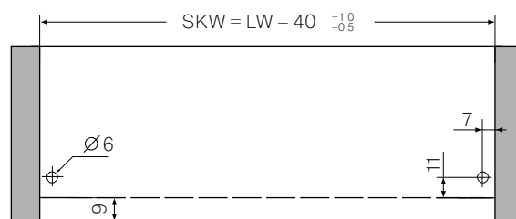
Задняя стенка ящика
