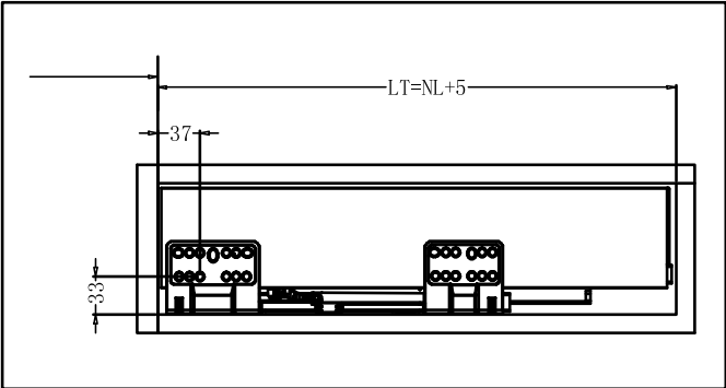
Установочные размеры ящика
