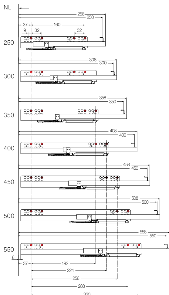
Присадка дна ящика с направляющими под штырь
