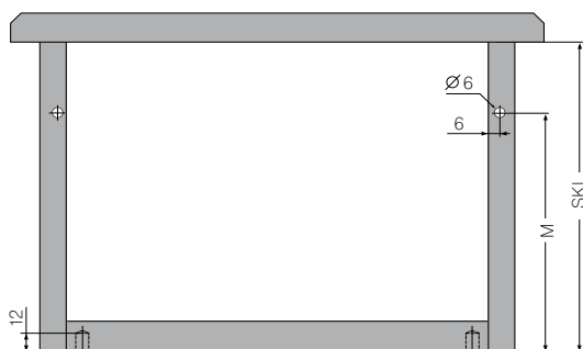
Присадка дна ящика с направляющими под штырь
